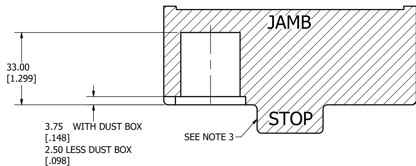
SECTION A-A
